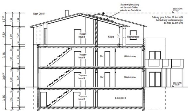
Querschnitt A-A Gebäude 1
